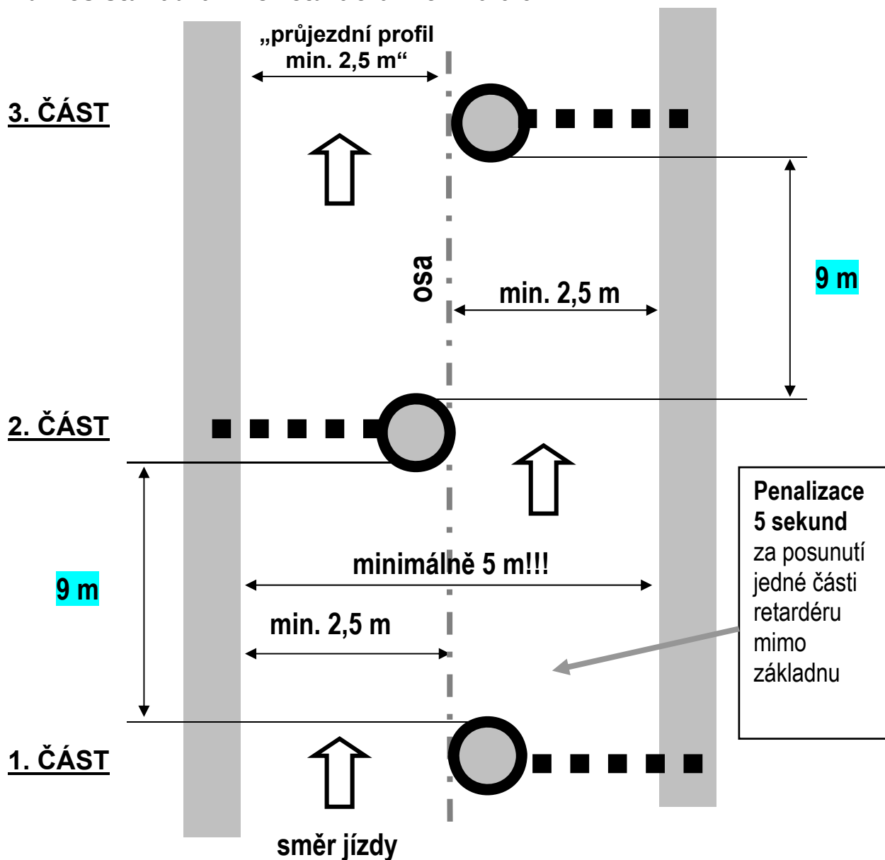
Příklad posunutí prvku ze základny v retardéru.
